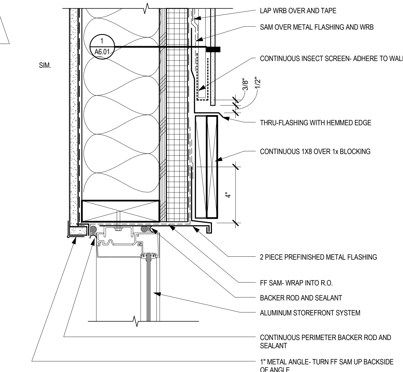
7 SF HEAD1 3" = 1'-0"
