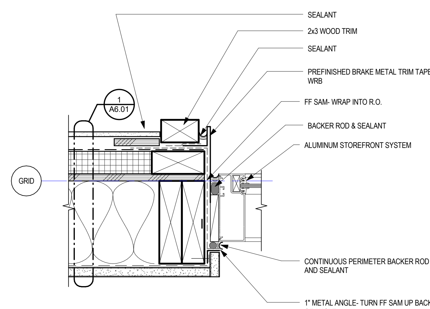
7 SF HEAD1 3" = 1'-0"
